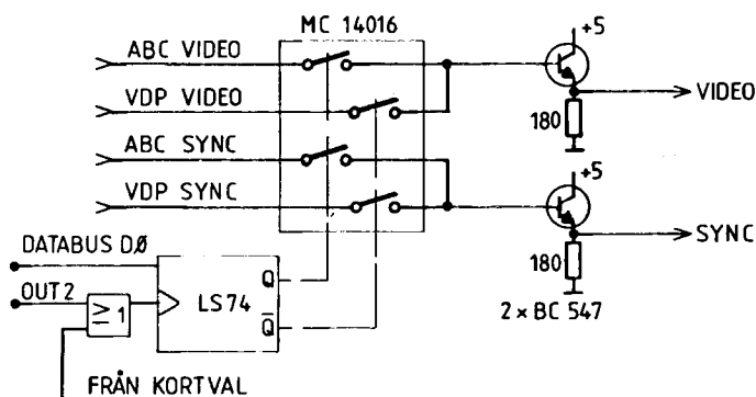
ABC-VDP VER.2 VIDEO-OMKOPPLARE
