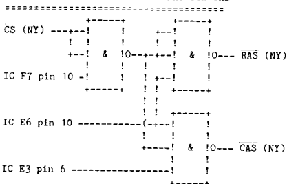
SCHEMA ÖVER INKOPPLINGEN AV RAS OCH CAS
