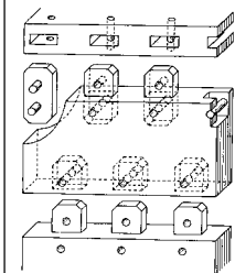
Tapp- och taphålsteknik.
